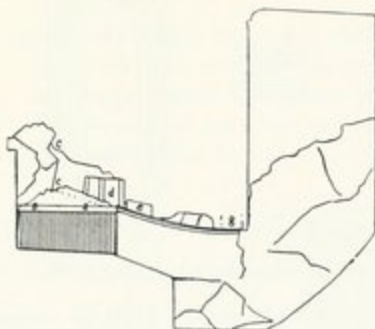
Fig. 333. — Profile.
