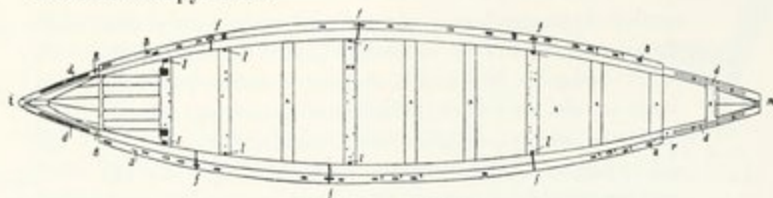
Fig. 311. — Deck plan.
