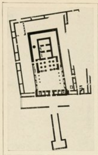
FIG. 444. — PLAN DU TEMPLE DE KALABCHÉH. (D'après Barsanti.)
