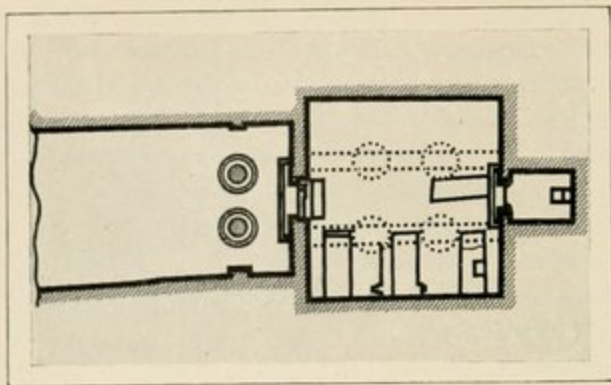
FIG. 186. — PLAN DE L'HYPOGÉE D'AMONI, A BÉNI-HASSAN. (D'après Newberry.)
