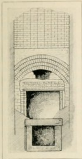
FIG. 67. — MASTABA A FOUR DE LA VI e DYNASTIE. (Dessin de Bourgoin, communiqué par la librairie A. Picard.)
