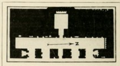
FIG. 254. — PLAN DU SPÉOS D'HARMHABI, A SILSILÉH.
