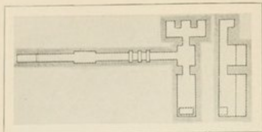
FIG. 76. — PLAN D'OUNAS. (Dessin d'après Maspero, communiqué par la librairie A. Picard.)
