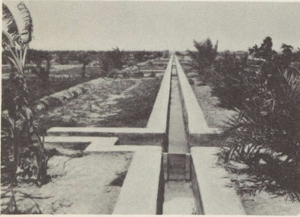
قناة عصرية للري مبنية بالكونكريت في بساتين تمر القطيف
