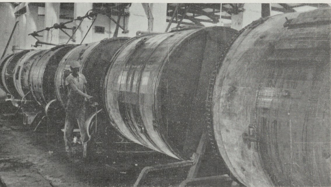
بعض آلات مصنع الدباغة في جدة
