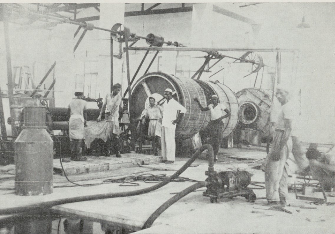
بعض آلات مصنع الدباغة في جدة
