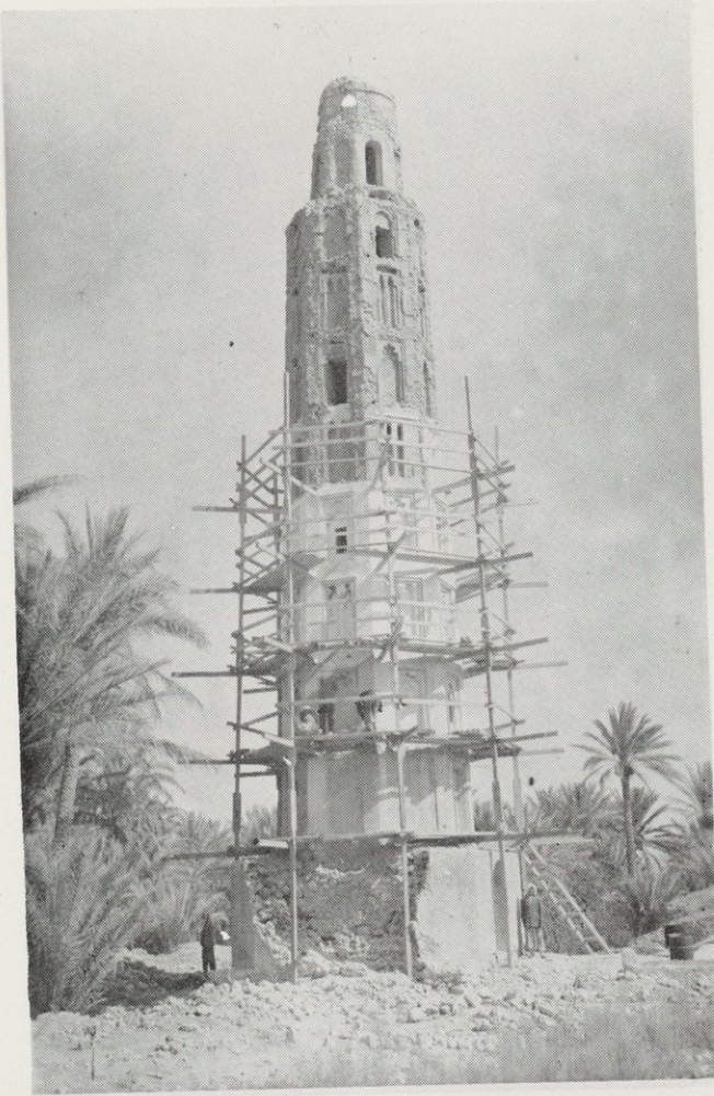
الشكل (٢٦) مئذنة عانة : من القرن الحادي عشر للميلاد وهي فريدة في شكلها . سحبت الصورة في اثناء عمليات الترميم
