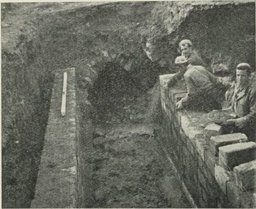
انشاء مجرى حديث وربطه بمجرى قديم في السليمانية
