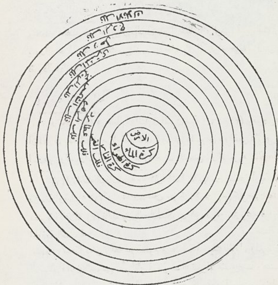
(ش - ١) النظام الشمسي البطليموسي
