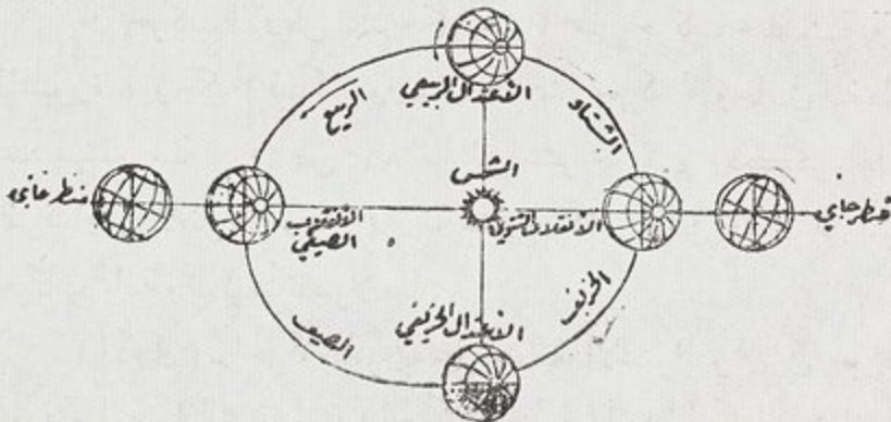
( ش هـ ) الأرض في الحركة السنوية حول مركز الشمس
