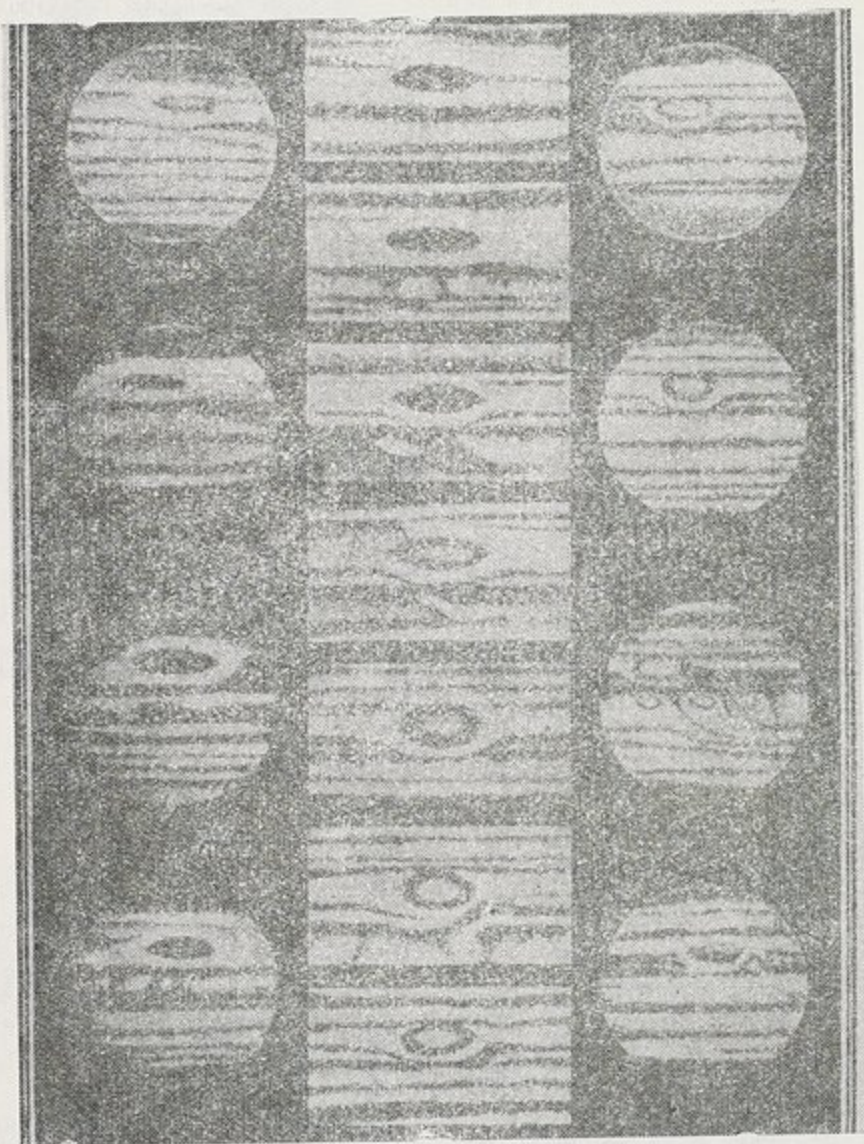
(ش ۱۲) المشتري ومناطقه وبقعه
