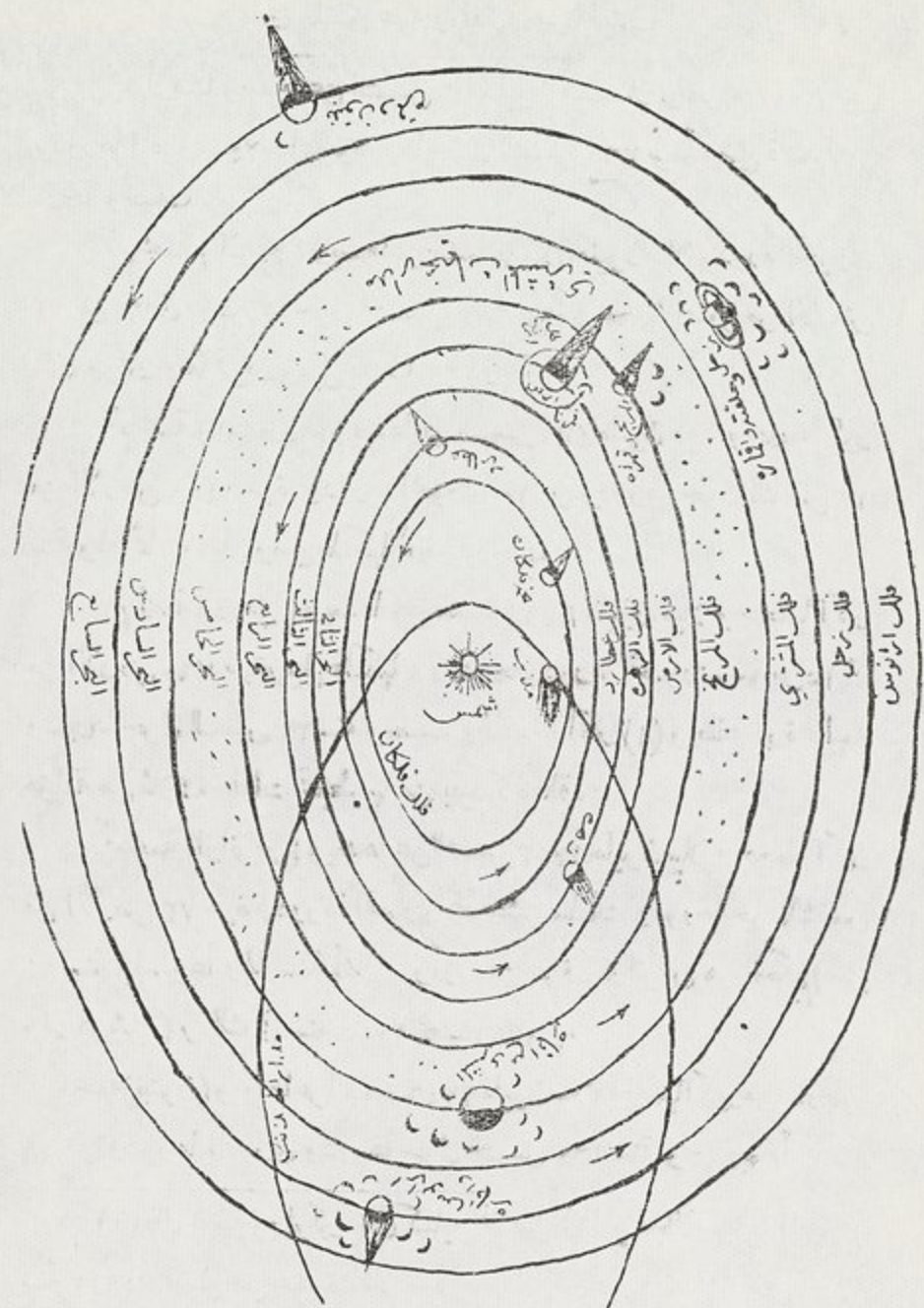
(ش - ٢) النظام الشمسي الكوبرنيكي
