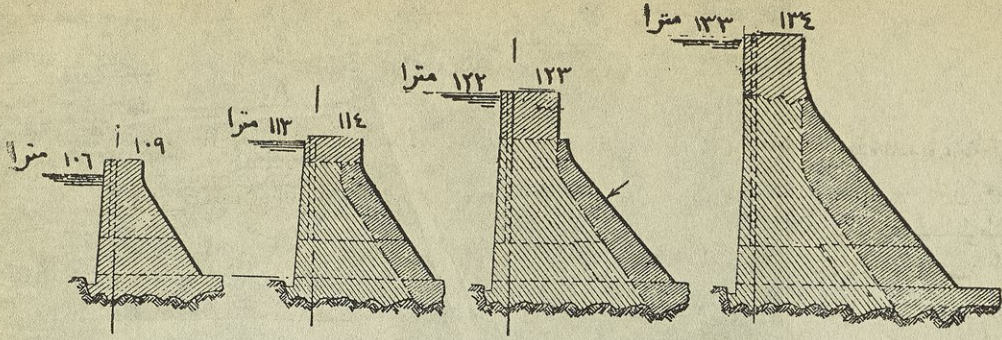
الحزان الاصلى ١٩٠٢ بعد التعلية الاولى ١٩١٢ بعد التعلية الثانية ١٩٣٣ التعلية الثالثة المقترحة ١٩٤٥
