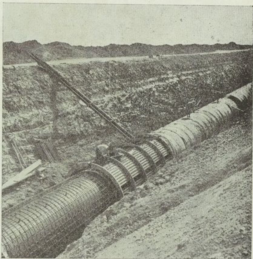
منظر آخر لعمليات انشاء المجاري
