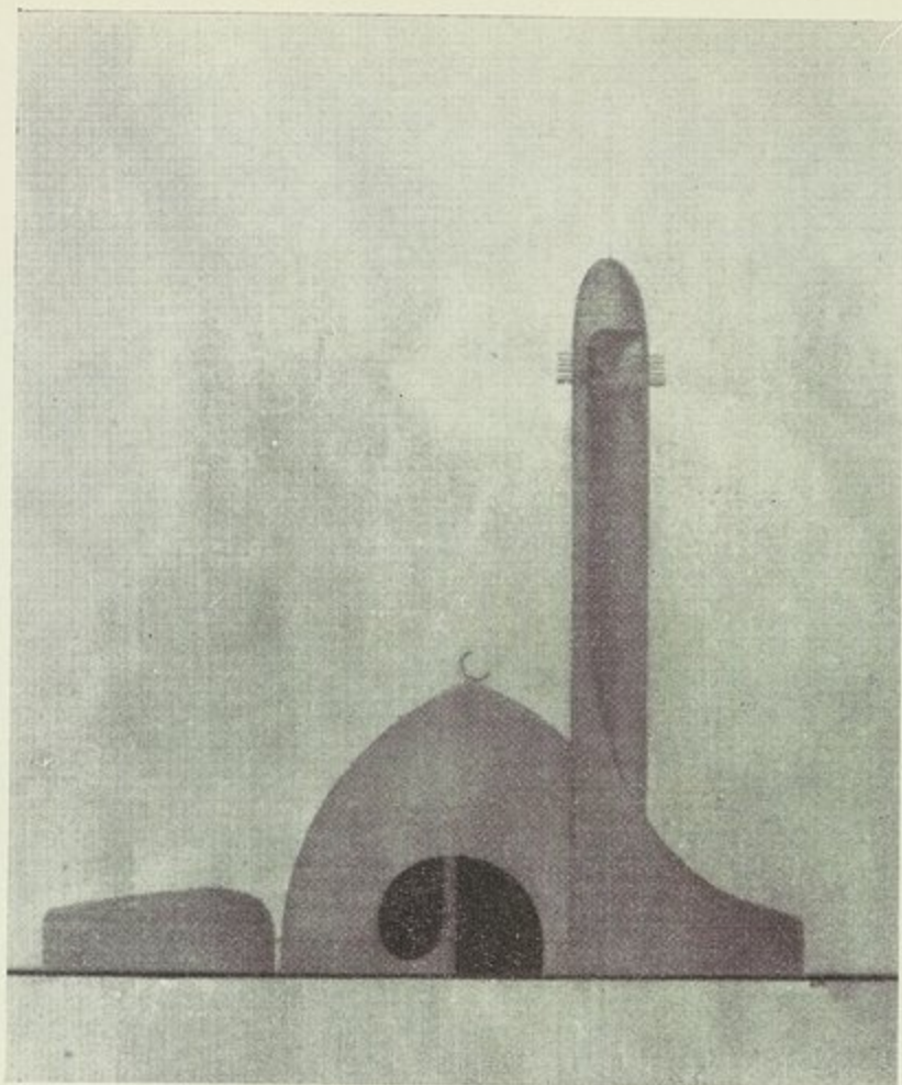
تصميم جامع ٠٠ في المركز المدني شرقي بغداد
