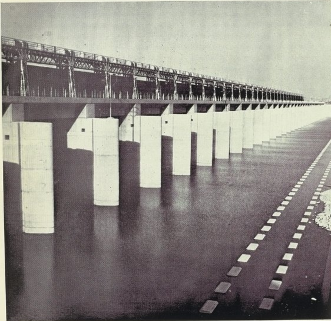
أحد منشآت الري الحديثة في الجمهورية العراقية مشروع الثرثار على دجلة
