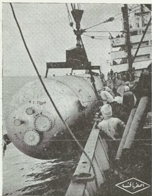
احدى وحدات الهايدر فورمر لتحسين نوع البنزين أثناء إنزالها الى الساحل في الدمام
