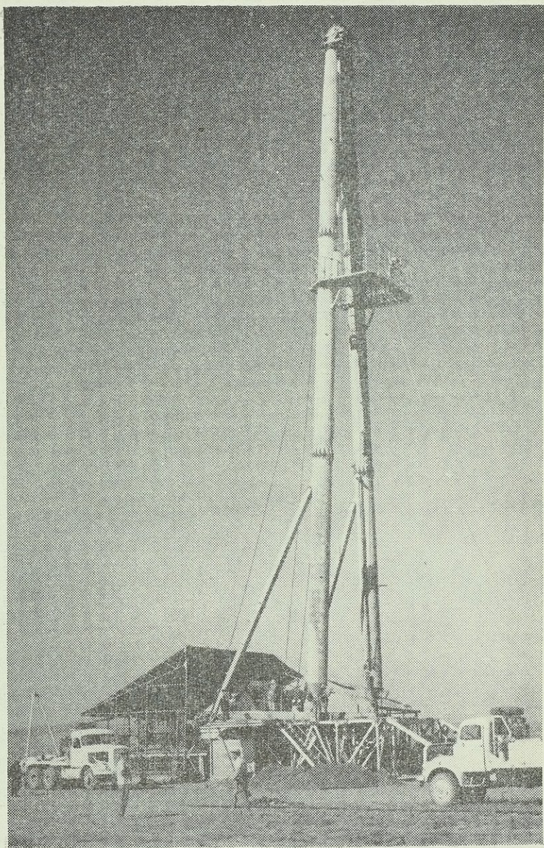
أحدث وأكبر آلة لاستخراج البترول نصبها شركة كونكورديا في الجزيرة وبدأت الحفر في أواخر آب
