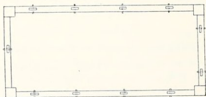
Fig. 12. — Cuve. Tenons du couvercle maintenus par des chevilles (41018).
