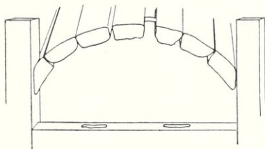
Fig. 9. — Assemblage du couvercle (41004, côté 1).
