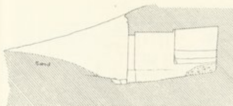
TOMB 9A—SECTION.
