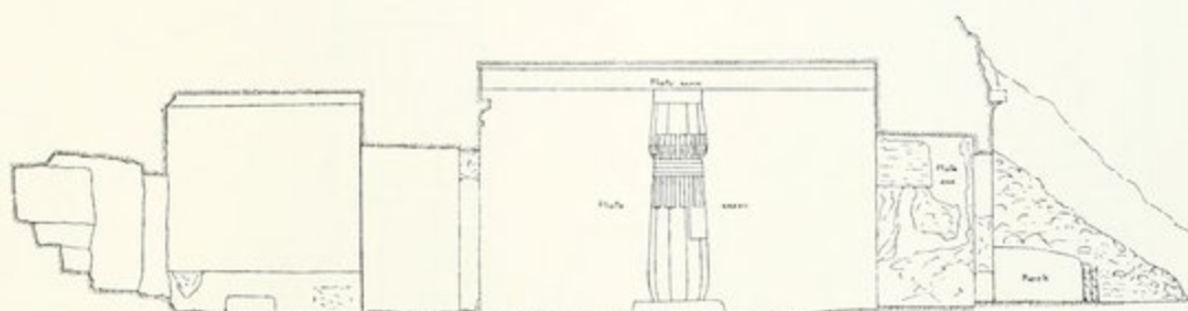
LONGITUDINAL SECTION.
