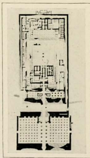
FIG. 235. — PLAN DU TEMPLE PRINCIPAL, A KARNAK. (Cliché Bêato.)
