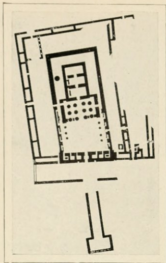
FIG. 444. — PLAN DU TEMPLE DE KALABCHÉH. (D'après Barsanti.)
