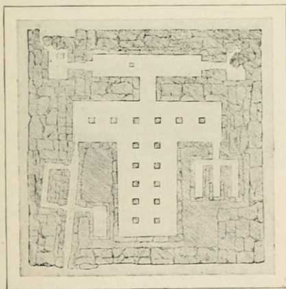
FIG. 85. — LE TEMPLE DU SPHINX. (D'après Mariette.)
