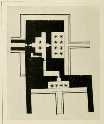
FIG. 81. — PLAN DE LA CHAPELLE DE SAHOURIYA. (D'après L. Borchardt.)
