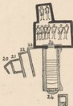
Scale, 1 : 250.
