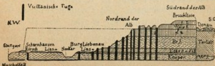
Schematischer Durchschnitt von Stuttgart bis nach Oberschwaben (NW nach SO) das Vulkangebiet von Donau. Aus Haas.
