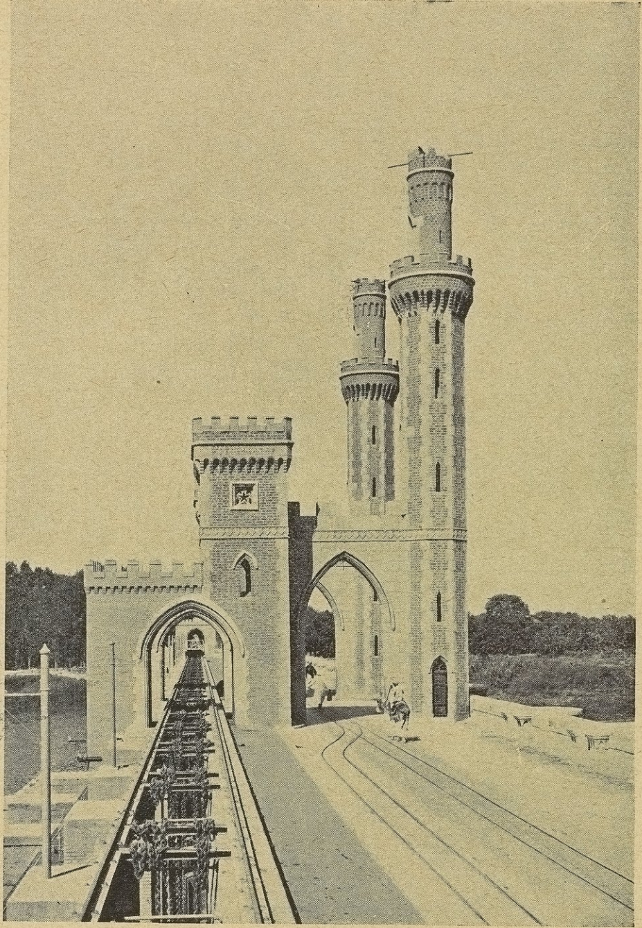
البنّاظر الجبّريّة بعد تقويّتها وتعدّلها
