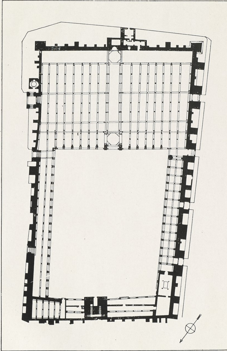
(شكل ٢) الرسم التخطيطي لمسجد القيروان
