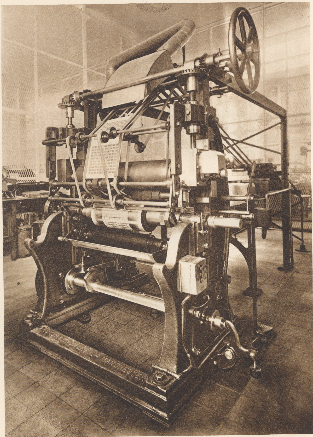
ماكينة للطباعة بطريقة الفوتوجرافير Photogravure Printing Machine
