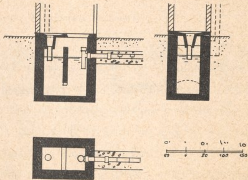
الشكل رقم ١٤ - تصميم المرحاض المائي .
