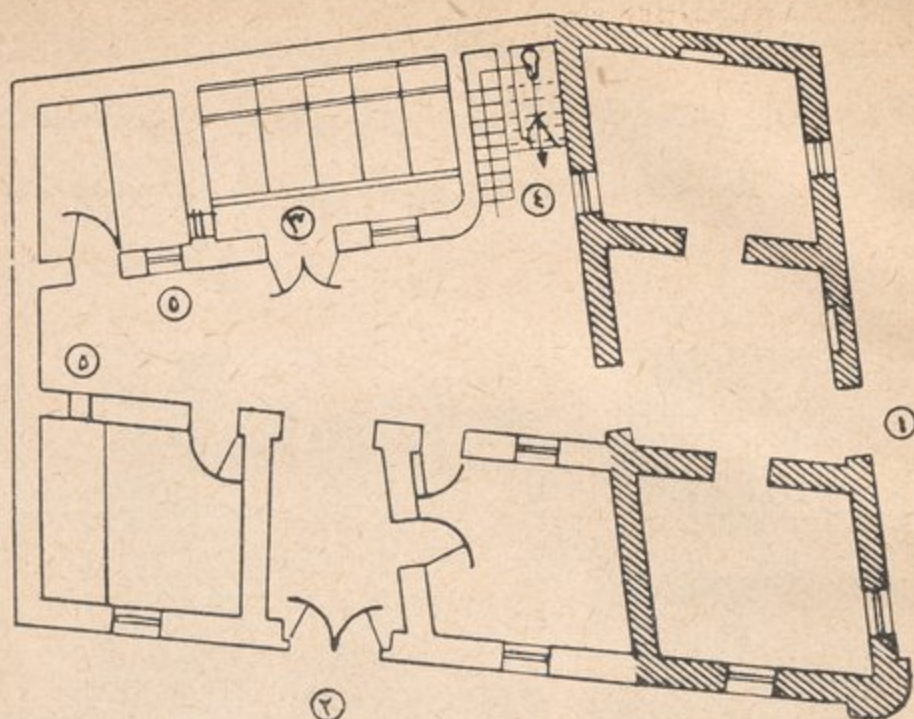
الشكل رقم ١ - تصميم مسكن ريفي في قرية فيشا الصغرى بمديرية المنوفية . إلى اليمين الجزء الأمامي من البناء وإلى اليسار الجزء الخلفي من البناء . ( ١ ) مدخل المسكن ( ٢ ) مدخل الحيوانات ( ٣ ) الحظيرة ( ٤ ) دورة المياه ( ٥ ) الحجرات الشوية ولها فتحات خارجية للفرن .
