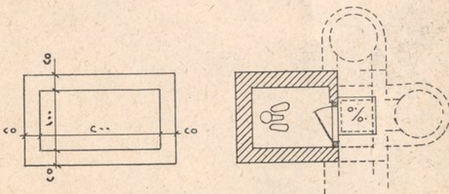
الشكل رقم ١٠ - تصميم مرحاض المجرور (البلدى).
