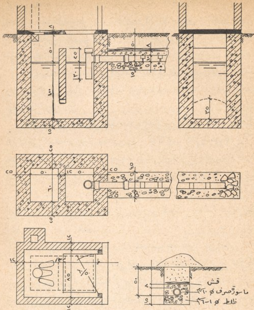
الشكل رقم ١٣ - تصميم المرحاض التحليلي .
