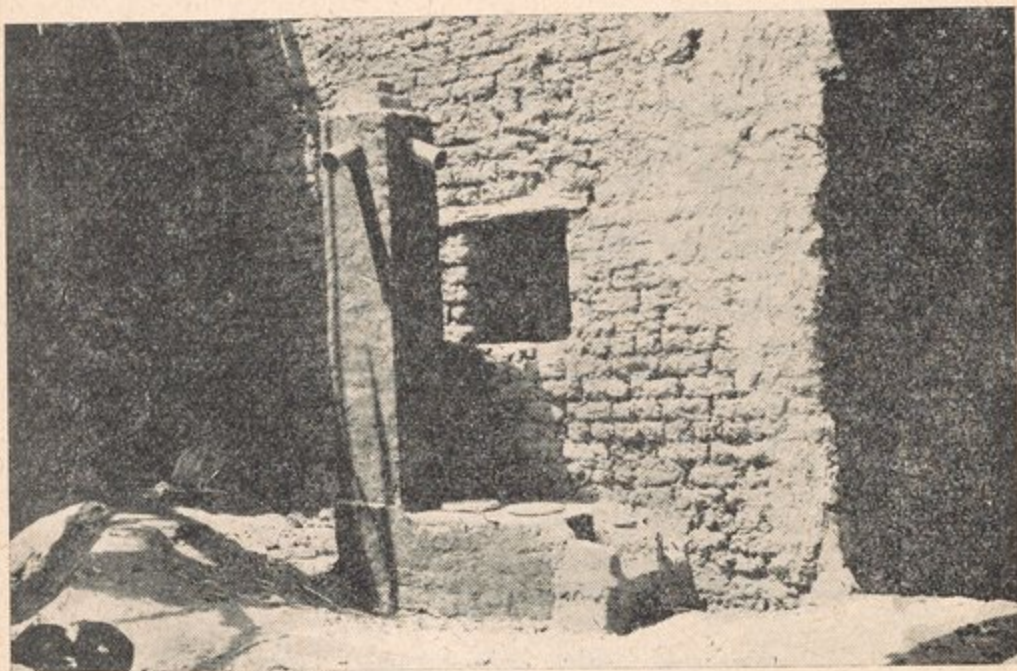
الصورة رقم ٢٠ - الموقد الريفي المحسن وقد تم بناؤه وأعد للاستعمال .
