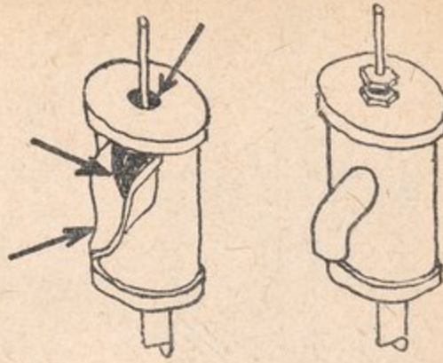
الشكل رقم ٧ : إلى اليسار طلمبة غير صحيحة : الفوهة أفقية مفتوحة . إلى اليمين طلمبة صحيحة : الفوهة مغطاة .
