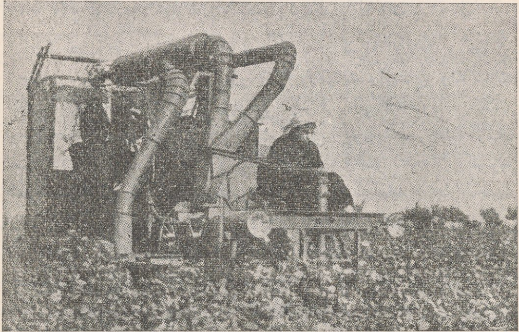
ماكينة حديثة لجنى القطن في الهند ( تملكها وتشغلها جمعية تعاونية زراعية متعددة الأغراض )
