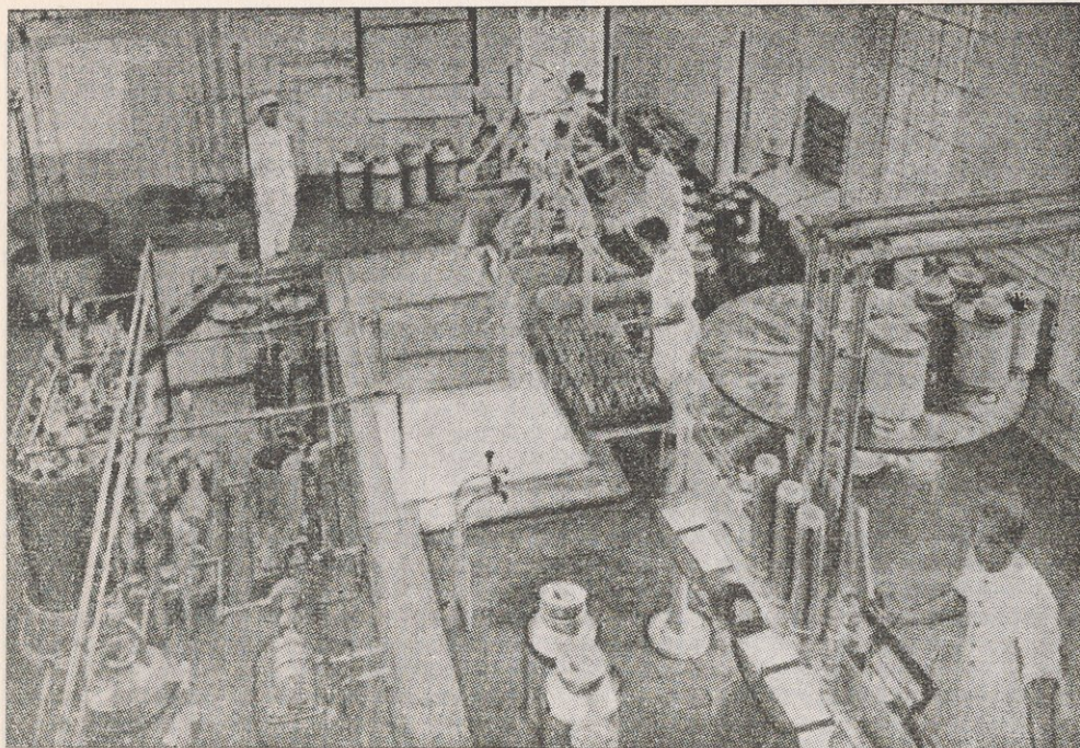
يوزن اللبن عند دخوله المعمل . وتقاس درجة نظافته ودسامته بالماكينات
