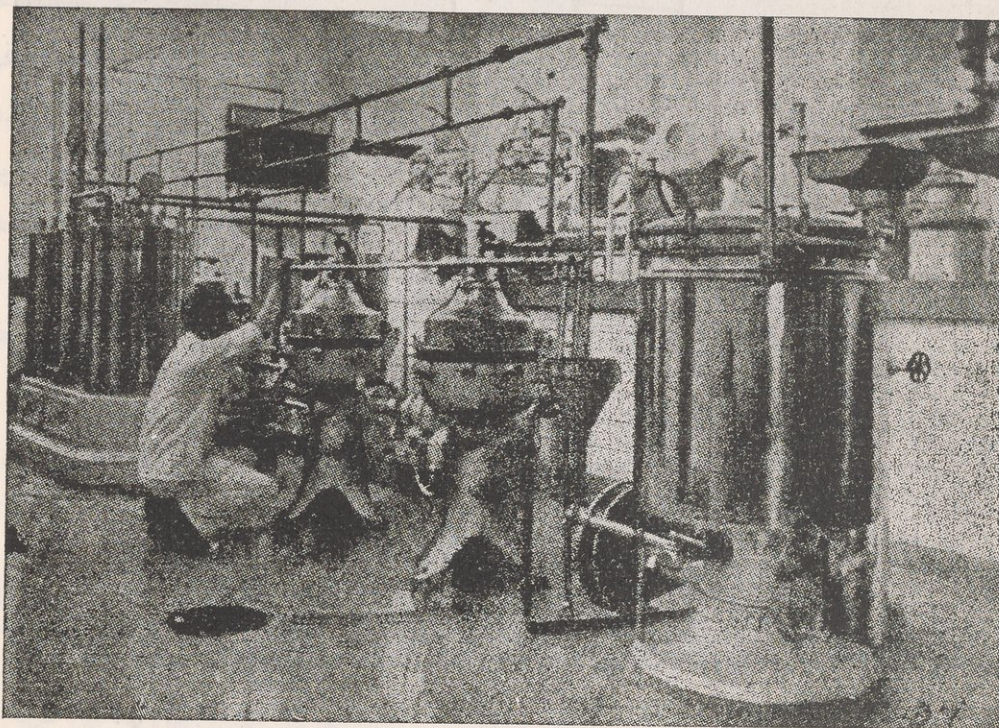
مجموعة من أحدث الآلات في معمل ألبان تعاوفى بالدانمارك .
