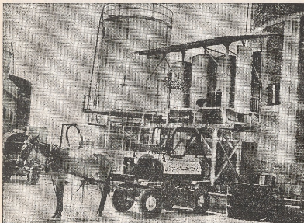
عربات التوزيع تمون من أنابيب الجمعية المذكورة
