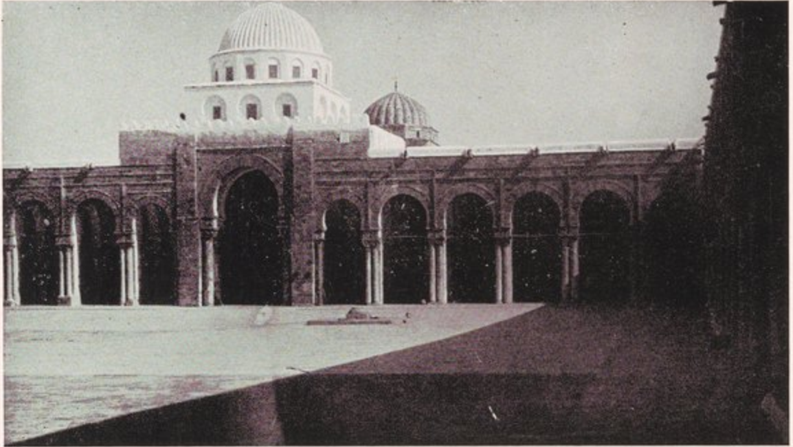
(شكل ٢٢) واجهة المجنبه القبليه من أعمال أحمد بن ابراهيم
