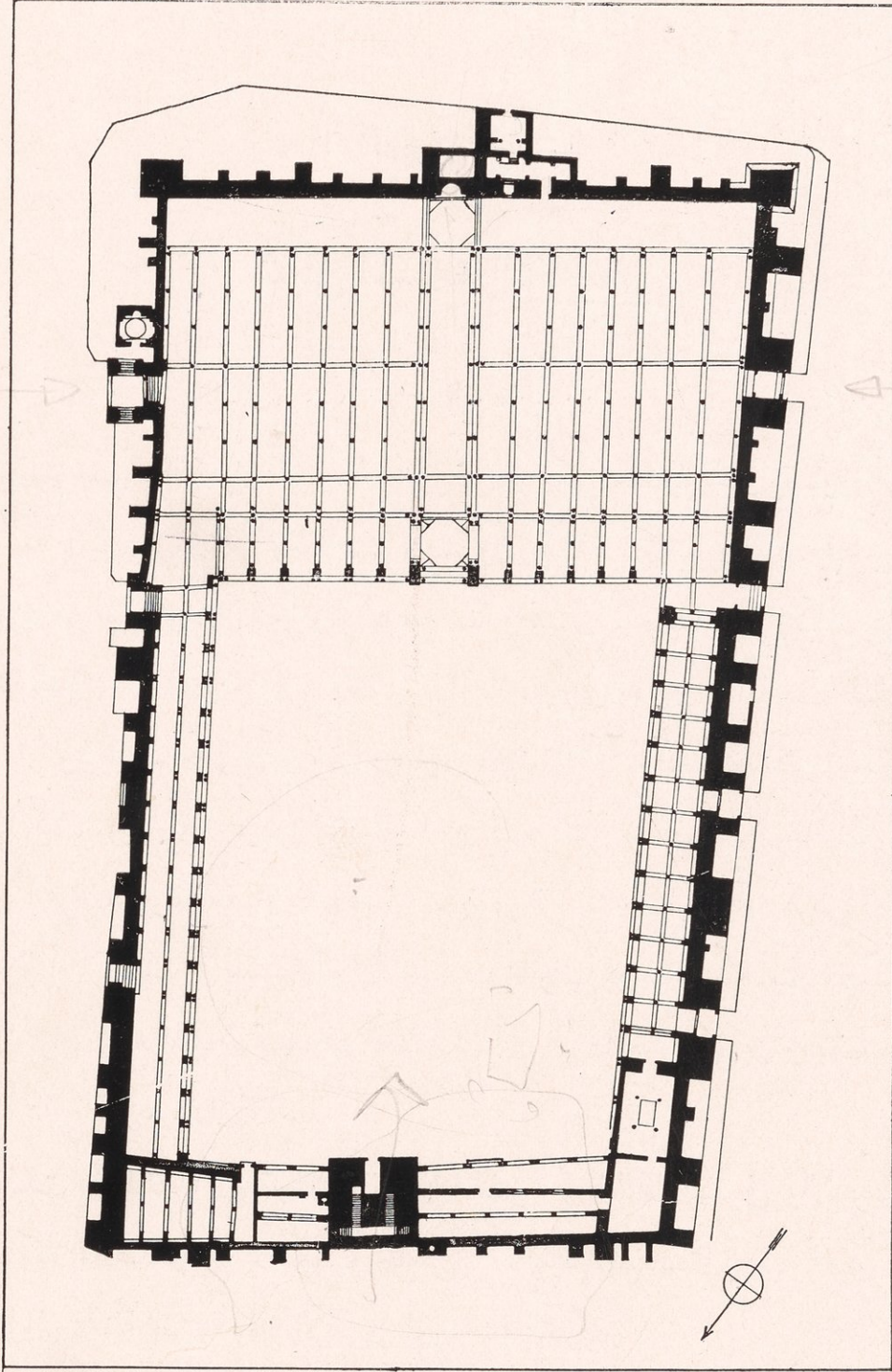
( شكل ٢ ) الرسم التخطيطى لمسجد القىروان
