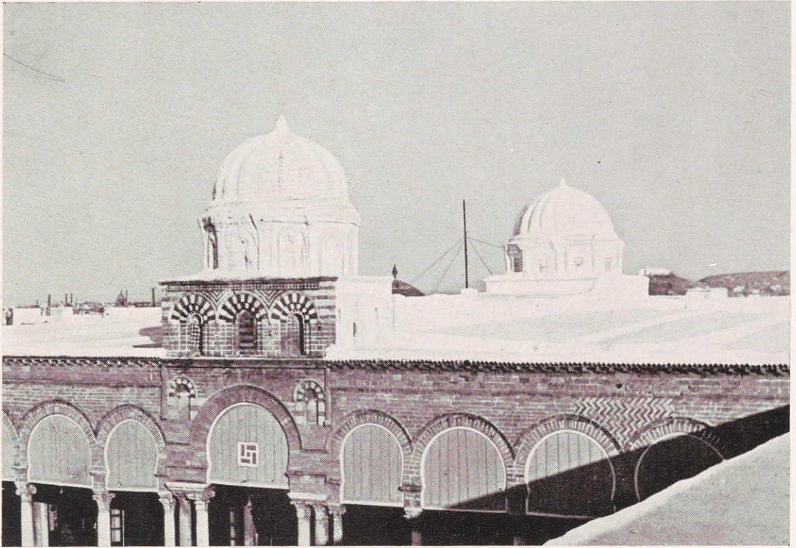
(شكل ٣٧) قبتا بيت الصلاة من مسجد الزيتونة بتونس
