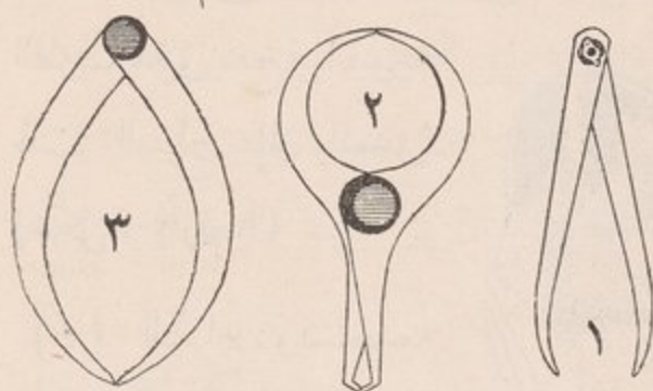
(شكل ٢٠٧) (١) الدوّارة المقصّية
