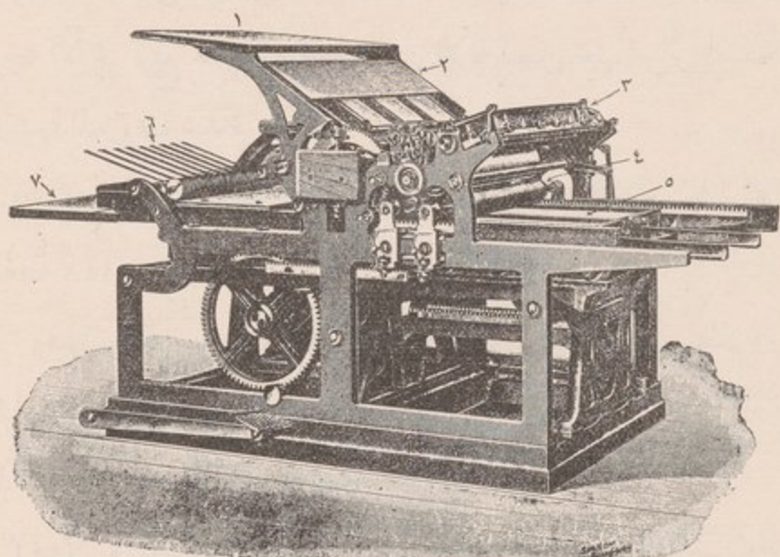
( شكل ٢٢٥ ) (١) رزمة الورق على استعداد لملحها الى حيث تقطع (٢) صحيفة من الورق في طريقها الى الطبع (٣) المحبرة تلوث اسطوانات الحبر تحتها (٤) الاسطوانة النظيفة فوق صحائف الحروف (٥) نحاسة ( الفورمة ) أو الصحيفة البيضاء فوق صحائف الحروف لا ينقصها إلا ضغط الاسطوانة عليها (٦) حمالة الورق المطبوع (الشراعة) (٧) رزمة الورق بعد طبعها ورقة ورقة .
