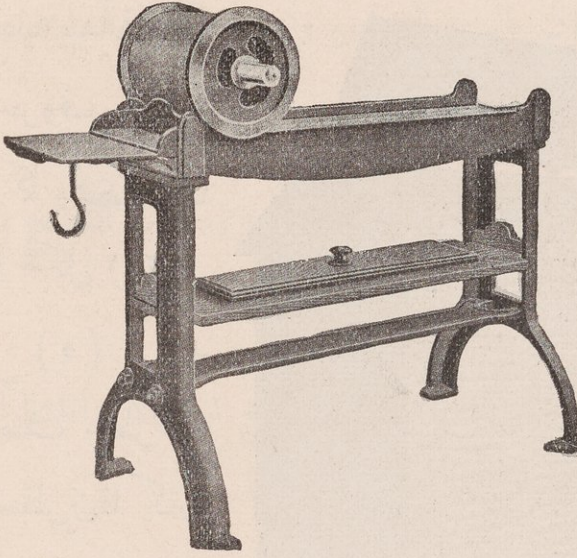
(شكل ٢٢٣) مطبعة التجارب
