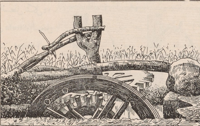
شكل (١٦) التابوت وأجزأؤه
