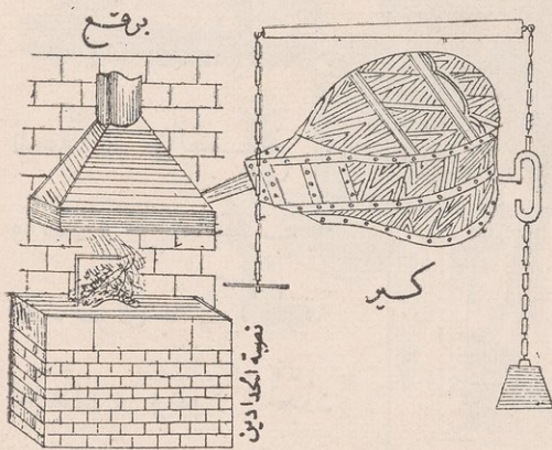
(شكل ٢٠٠) منصّب الحداد وأجزاؤه
