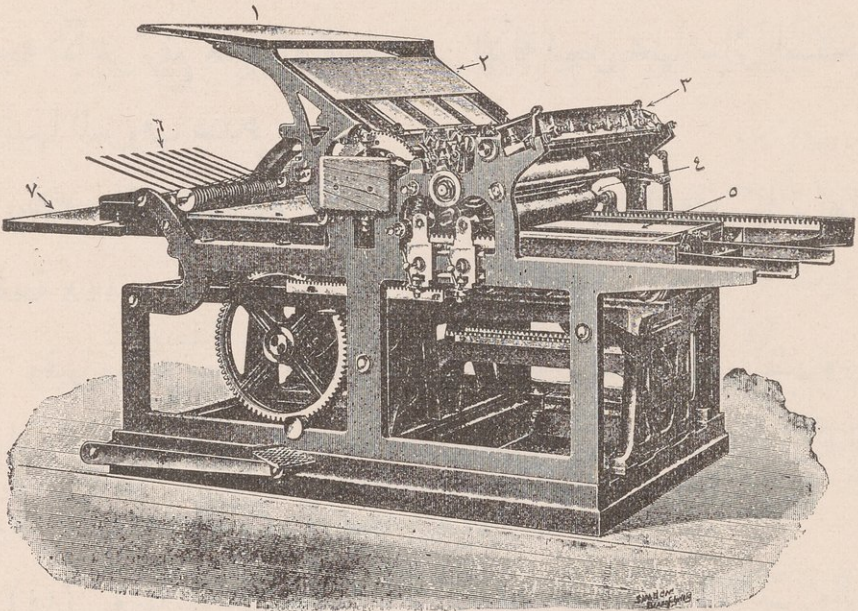
( شكل ٢٢٥ ) (١) رزمة الورق على استعداد لملئها الى حيث تطبع (٢) صحيفة من الورق في طريقها الى الطبع (٣) الحبرة تلوث اسطوانات الحبر تحتها (٤) الاسطوانة النظيفة فوق صحائف الحروف (٥) نحاسة (الفورمة) أو الصحيفة البيضاء فوق صحائف الحروف لا ينقصها إلا ضغط الاسطوانة عليها (٦) سمالة الورق المطبوع (الشراعة) (٧) رزمة الورق بعد طبعها ورقة ورقة .
