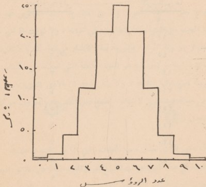
(شكل ١) يمثل هذا المنحني كثرة ظهور الرؤوس حين ترمي ١٠ قطع من النقود ١٠٢٤ مرة
