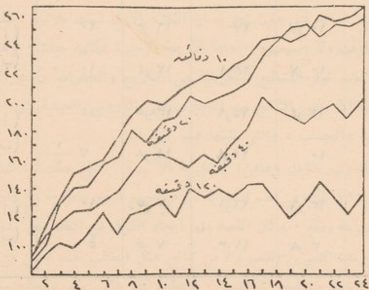
(شكل ٣٥) منحنيات التقدم اخذت من تجربة كان فيها التمرين في اربع حصص مختلفة
