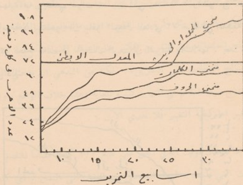
(شكل ٣٢) تبين هذه المنحنيات تعلم الاحرف والكلمات والجمل في البرق
