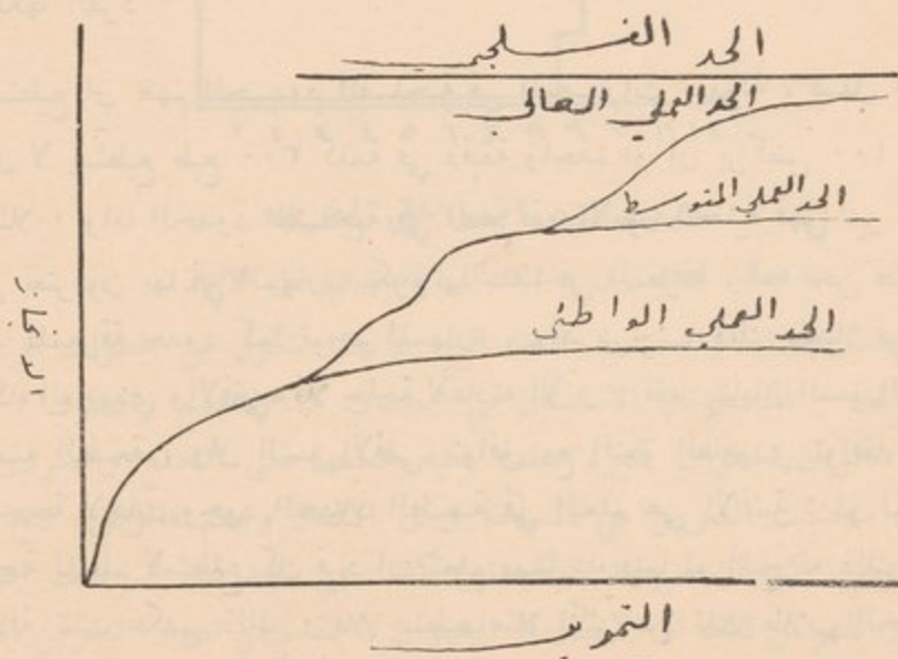
(شكل ٣٤) يبين هذا المنحنى العلاقة بين الحد العملي والحد الفلسفي
