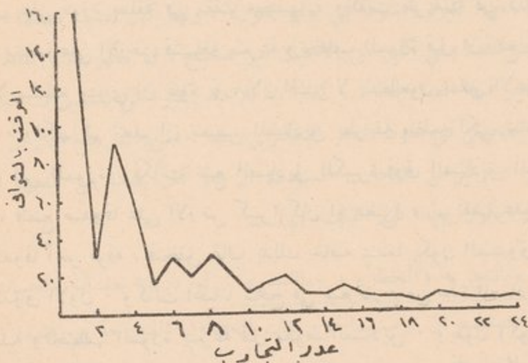
(شكل ٢٨) منحنى تعلم القطعة . «الوقت» يعني الثواني التي احتاجتها للتخلص من صندوق الالغاز .
