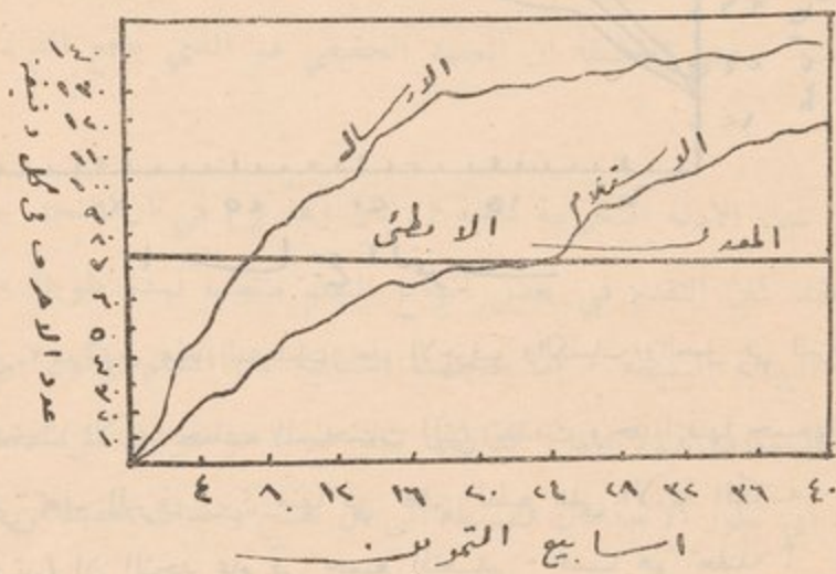
(شكل ٣١) تبين هذه المنحنيات التقدم في ارسال البرقيات واستلامها
