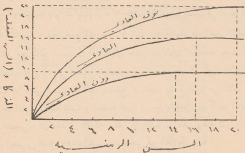
(شكل ٢٣) تبين هذه المنحنيات نمو الذكاء منذ الولادة حتى النضوج
