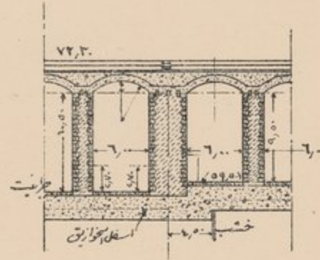
قطاع طولی فی الموصله بین فتحات ٥٨,٥٠ و ٥٩,٥٠ - مقياس الرسم ٤٠٠:١
