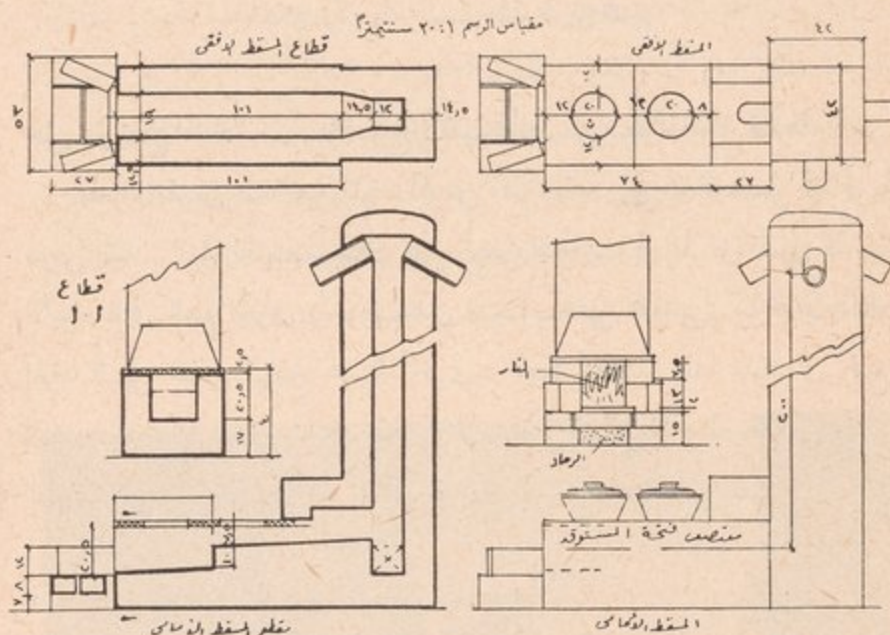
الشكل رقم ١٦ - تصميم الموقد الريفي المحسن
