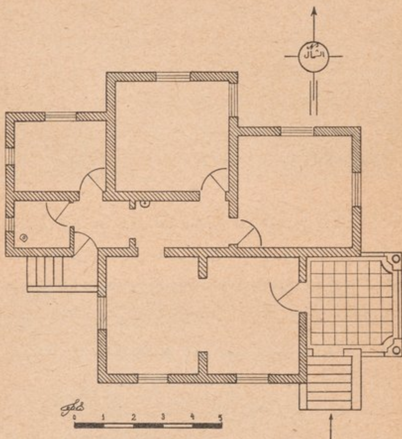
الشكل رقم ٢ - تصميم المسكن السابق .
