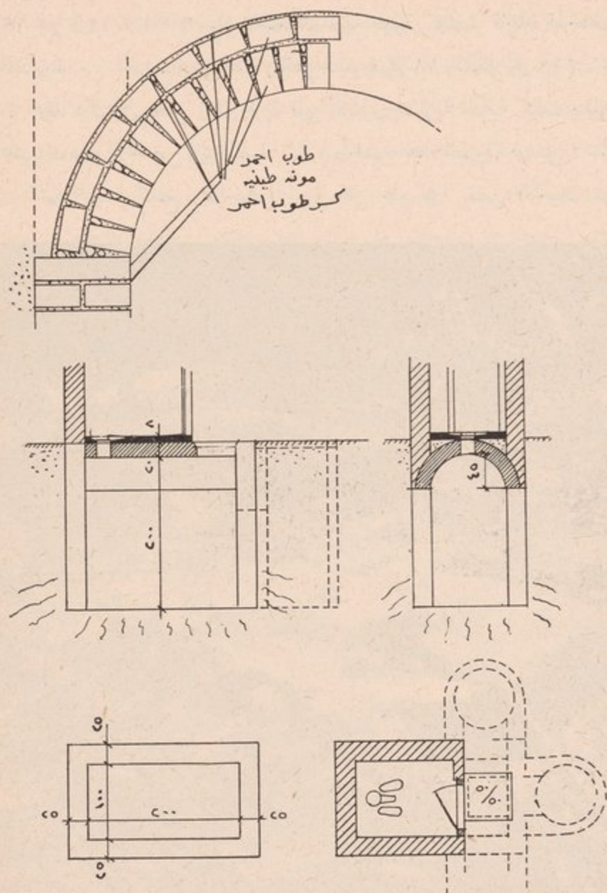
الشكل رقم ١٠ - تصميم مرحاض المجرور (البلدى).
