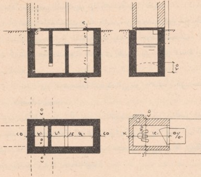
الشكل رقم ١١ - تصميم المرحاض ذى الخوض التحليلي .
