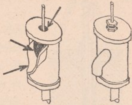
الشكل رقم ٧: إلى اليسار طلمبة غير صحية: الفوهة أفقية مفتوحة . إلى اليمين طلمبة صحية: الفوهة مغطاة.
