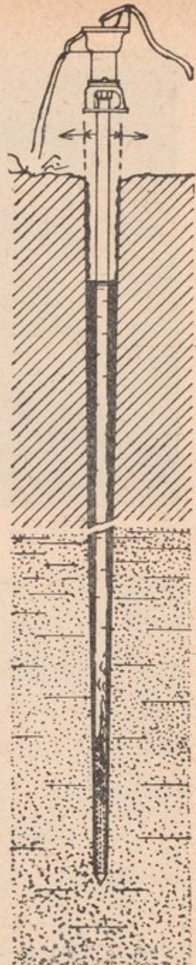
الشكل رقم ٥ - طلمبة بغير قاعدة تكون حول أنبوبها فراغ ناتج عن الاهتزاز وأدى إلى رشح الماء القذر وتلوث المياه الجوفية.
