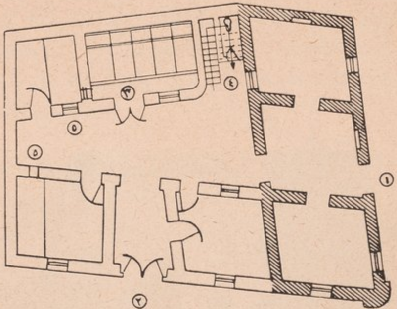
الشكل رقم ١ - تصميم مسكن ريفى فى قرية فيشا الصغرى بمديرية المنوفية . إلى اليمين الجزء الأمامى من البناء وإلى اليسار الجزء الخلفى من البناء . ( ١ ) مدخل المسكن ( ٢ ) مدخل الحيوانات ( ٣ ) الحظيرة ( ٤ ) دورة المياه ( ٥ ) الحجرات الشتوية ولها فتحات خارجية للفرن .
