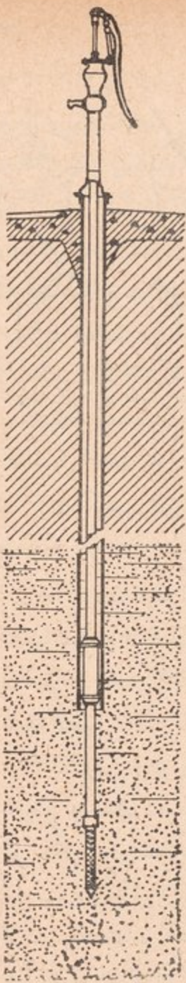
الشكل رقم ٦ - طلمبة أسطوانتها العاملة نازلة في الأنبوبة الخارجية ومغمورة في المياه الجوفية .
