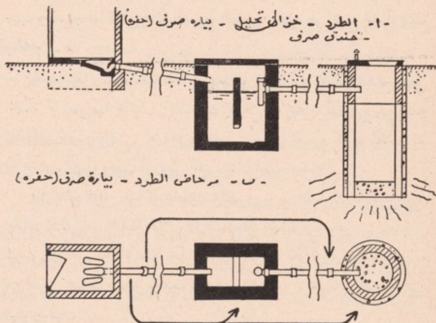
الشكل رقم ١٥ - تصميم مرحاض الطرد .
