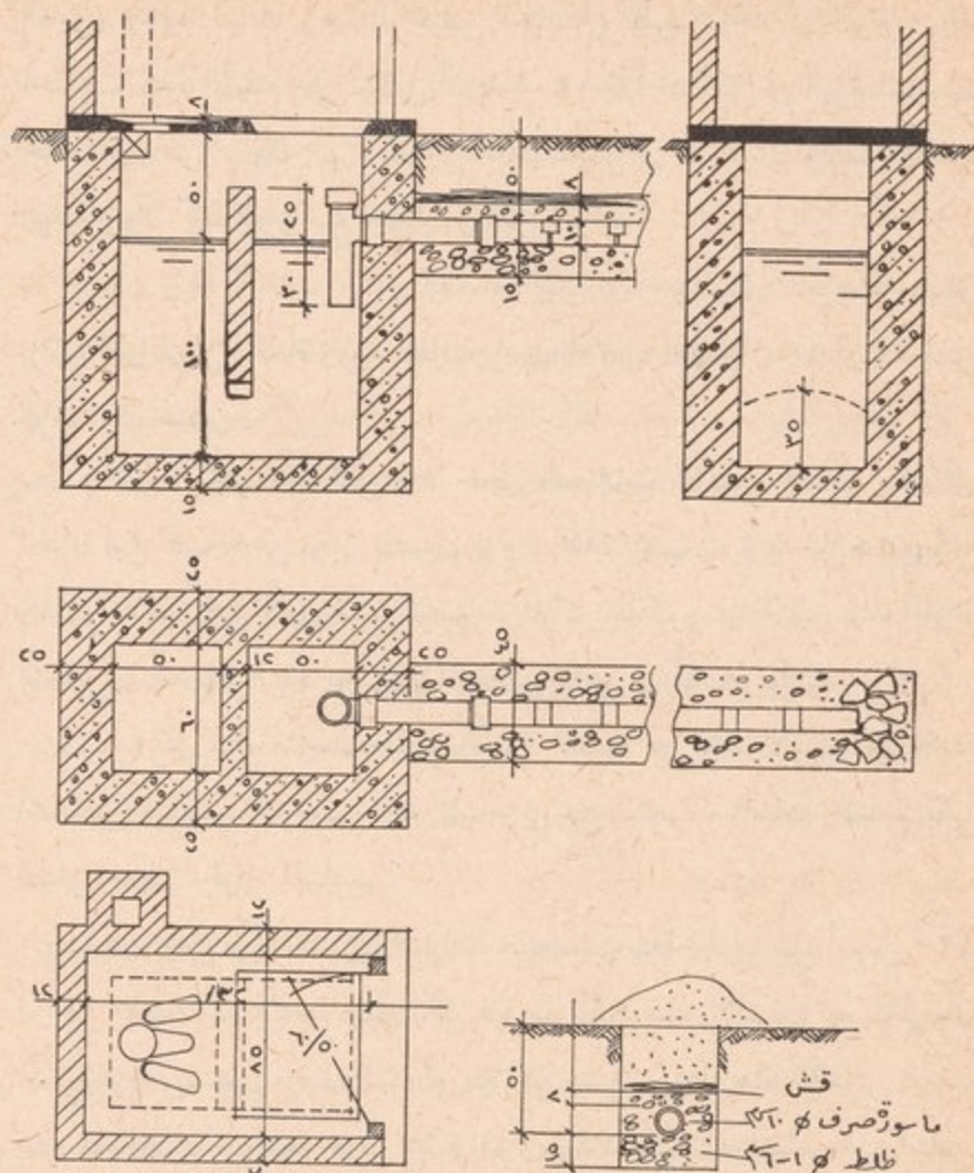
الشكل رقم ١٣ - تصميم المرحاض التحليلي .
