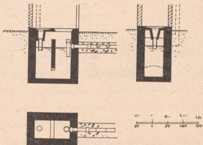
الشكل رقم ١٤ - تصميم المرحاض المائي .
