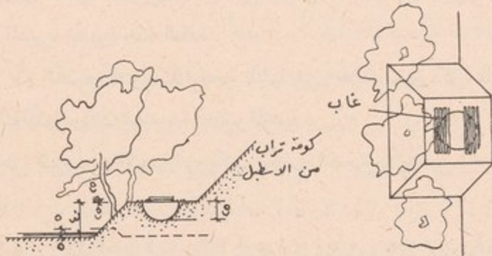
الشكل رقم ١٢ - تصميم مرحاض الحقل .
