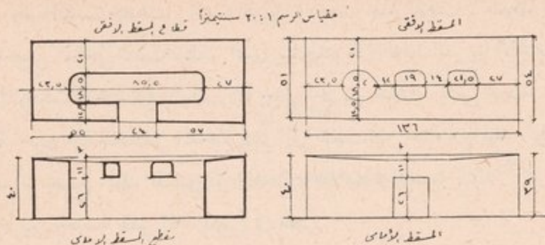
الشكل رقم ١٧ - تصميم الموقد الريفي القديم .
