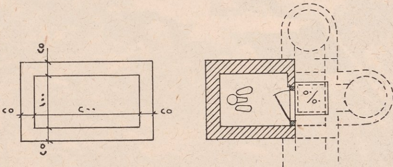
الشكل رقم ١٠ - تصميم مراحض المجرور (البلدي).
