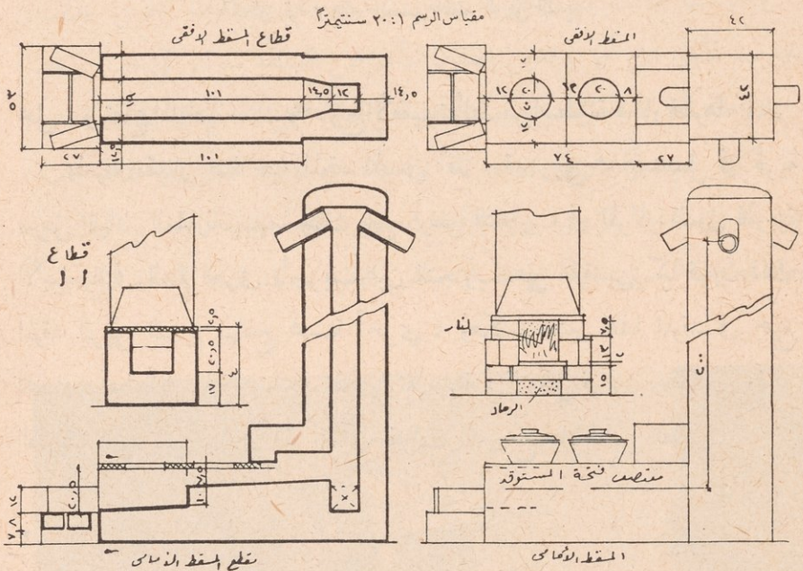
الشكل رقم ١٦ - تصميم الموقد الريفي المحسن
