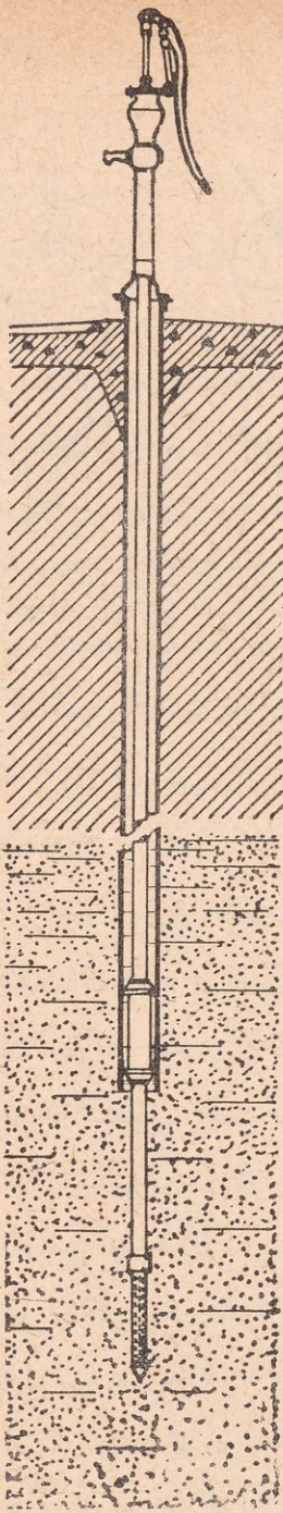
الشكل رقم ٦ - طلمبة اسطوانتها العاملة نازلة في الأنوبة الخارجية ومغمورة في المياه الجوفية .
