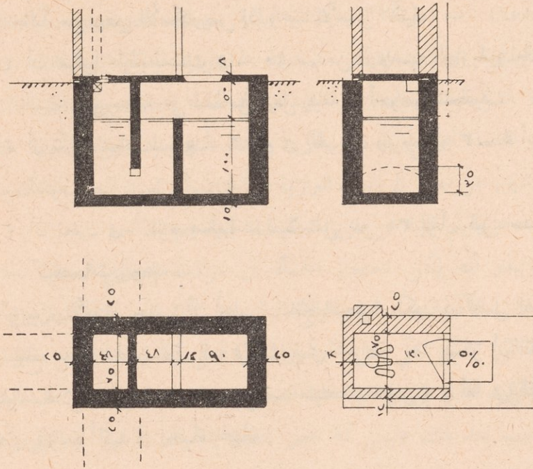
الشكل رقم ١١ - تصميم المرحاض ذى الحوض التحليلي .
