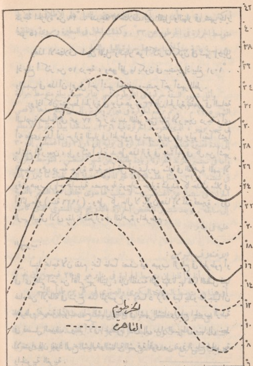
( شكل ٣٨ ) رسم بيان للنهاية الكبرى والصغرى ومتوسط الحرارة في كل من القاهرة والحارطوم
