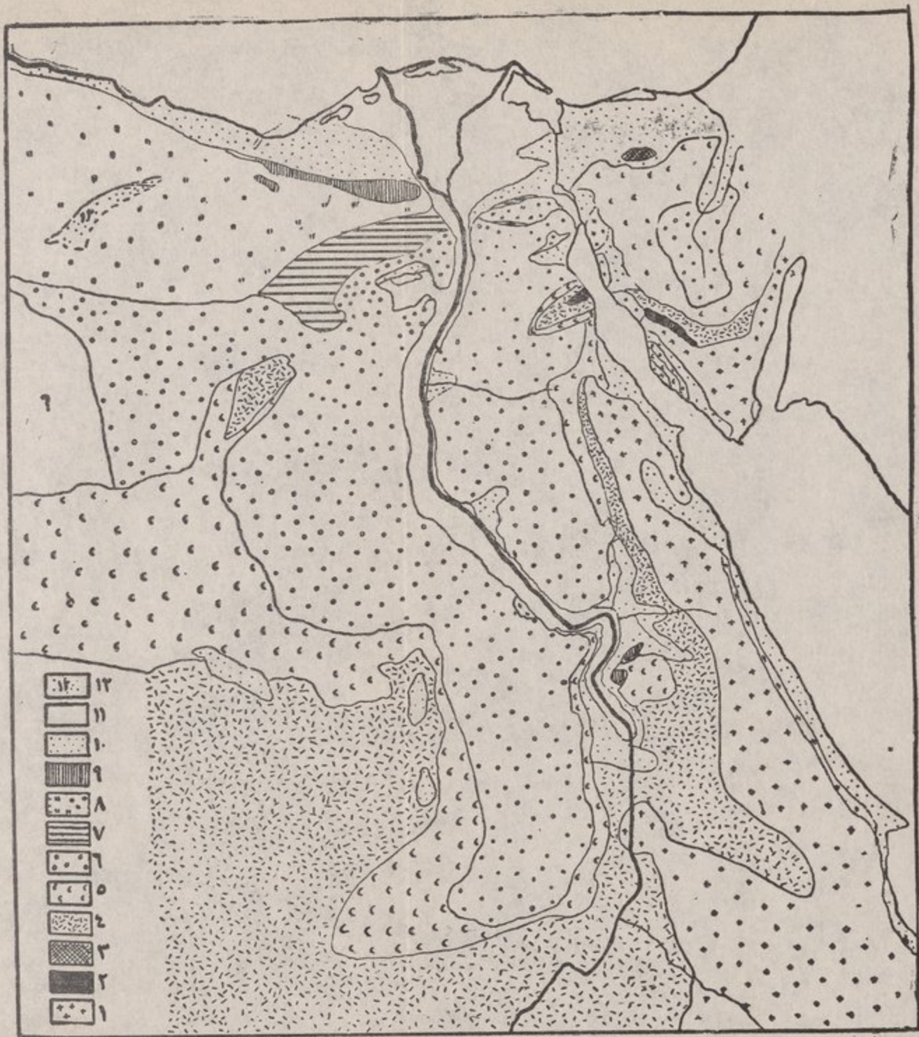
(شكل ١٩) خريطة جيولوجية للقطر المصري
