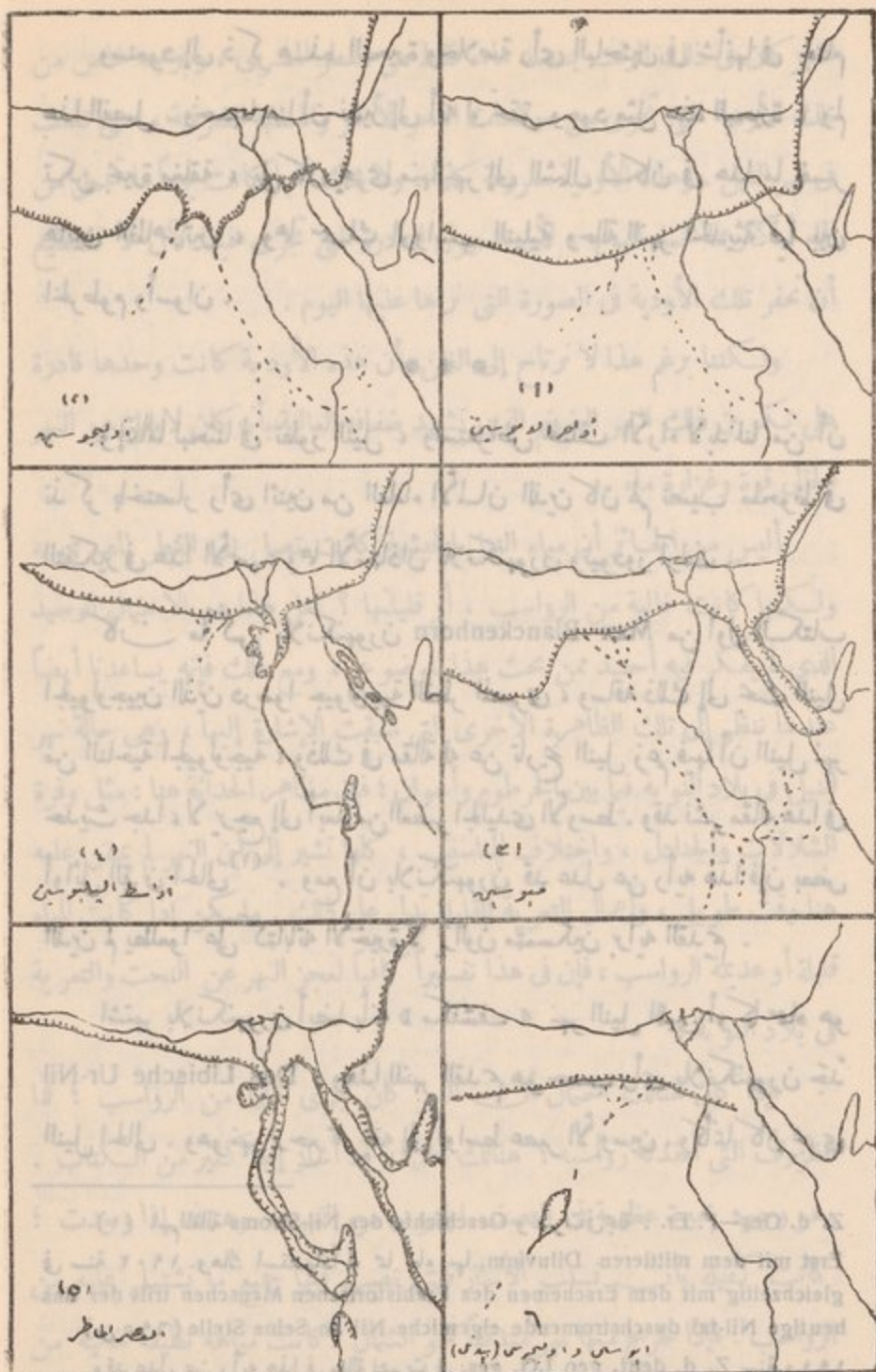
(شكل ٢٨) النيل الليبي كما تصوره بلانكنهورن (١ - ٥) وبيدزل (٦)
