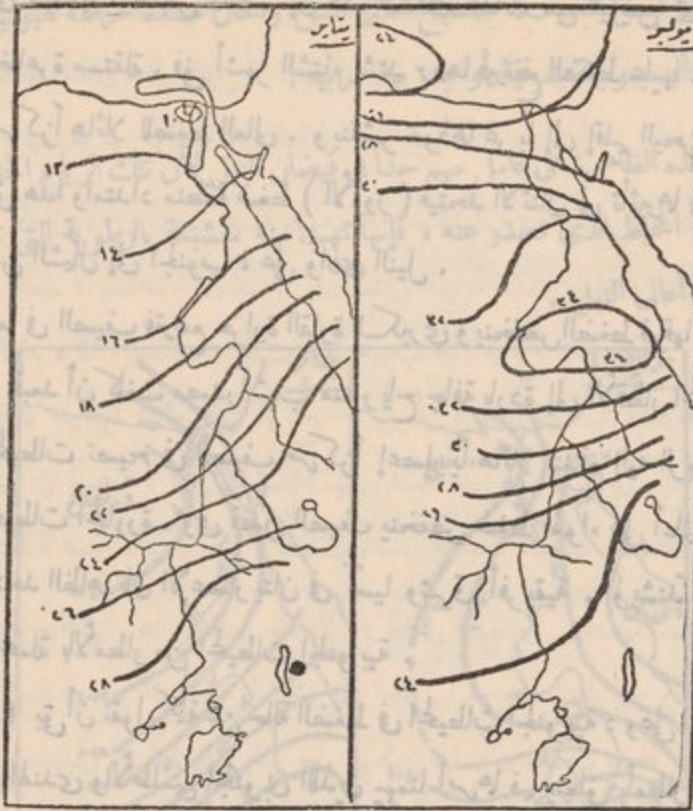
( شكل ٣٤ ) توزيع الحرارة في حوض النيل في شهرى بنابر ويوليو
