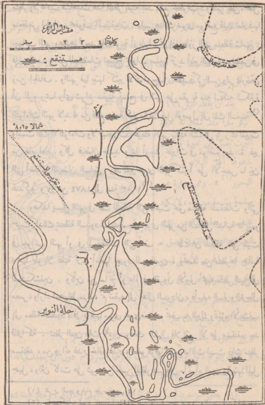
(شكل ٨) بحر الجبل في منطقة المستنقعات
