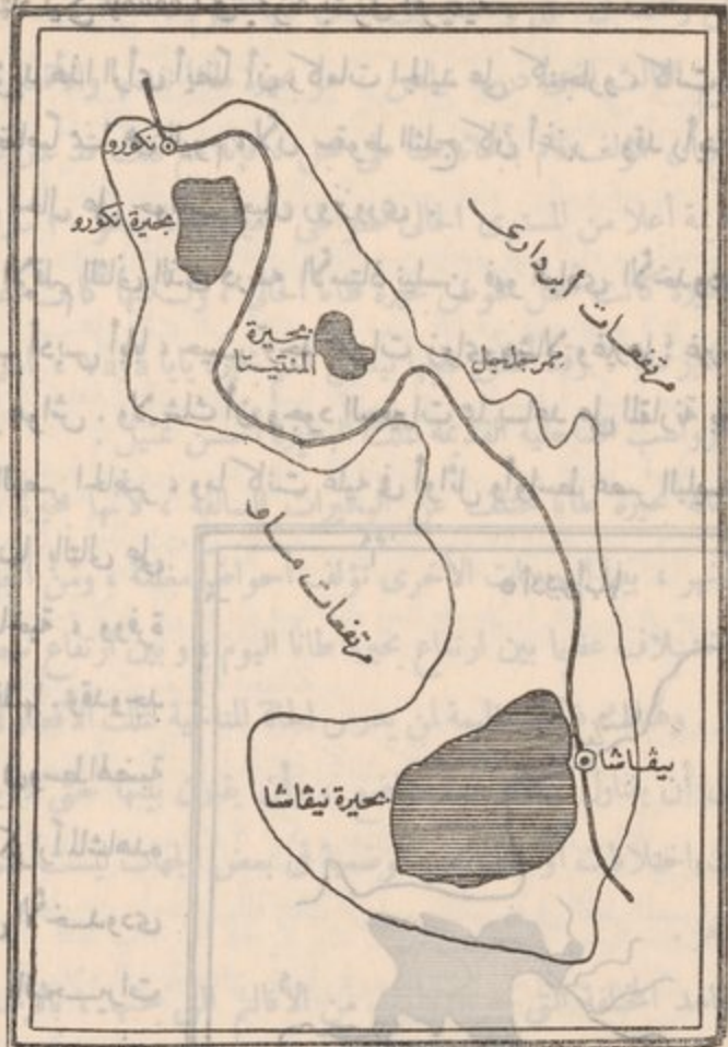
(شكل ٢٦) الحوض الأخدودي في كينا
