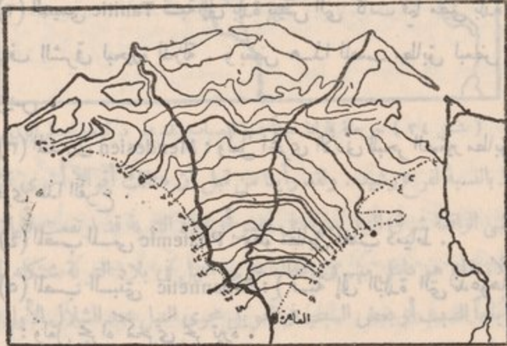
( شكل ٣١ ) خريطة الدلتا مبينا بها خطوط الارتفاع
