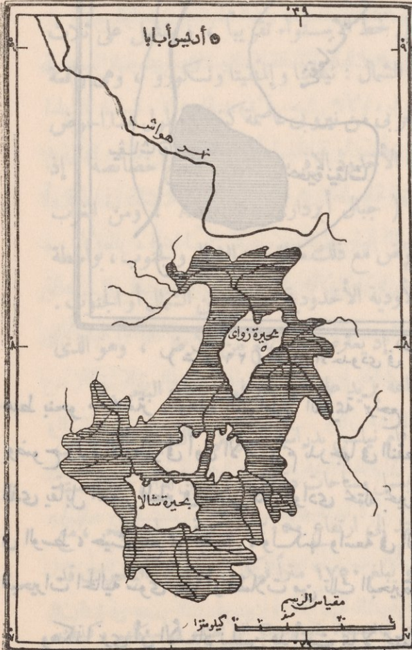
( شكل ٢٧ ) الحوض الأخدودى فى جنوب الحبشة
