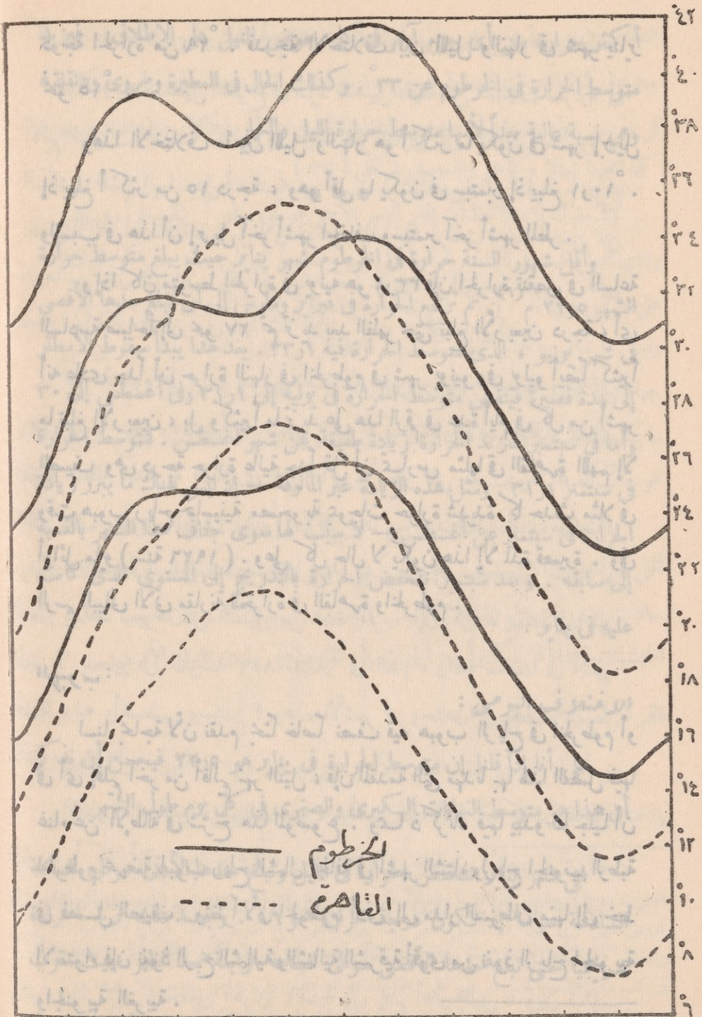
( شكل ٣٨ ) رسم بيان للنهاية الكبرى والصغرى ومتوسط الحرارة في كل من القاهرة والحرطوم
