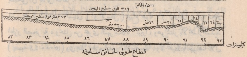
(شكل ١٥ و ١٦) خريطة وقطاع طولى لخائف سبلوق
