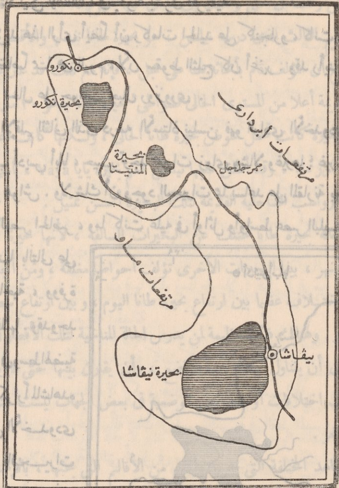
(شكل ٢٦) الحوض الأخدودي في كينيا
