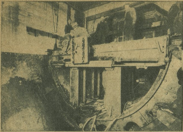
الى اليسار : منظر قطاعي من النفق بين عظم بنائه وقد رسمت هذه الصورة أثناء تشييده
