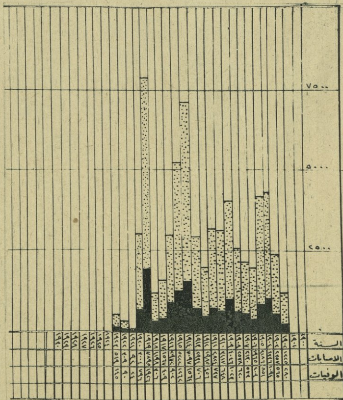
يبين هذا الرسم البياني عدد الاصابات والوفيات بالجدري في كل سنة من سنة ١٩٠٢ الى سنة ١٩٢٣
