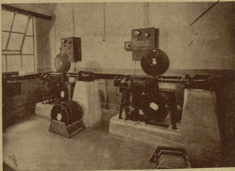
آلة التقاط الصوت وتسجيله على الاسطوانات في شركة « متروجلديون ماير »
