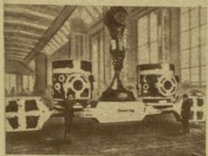
أكبر مغناطيس في العالم حجر المغناطيس الموجود في معامل كروب بألمانيا وقطره ١٥٠٠ مليمتر وهو يحمل ثقل قدره ٧٥ ألف كيلوجرام من الحديد
