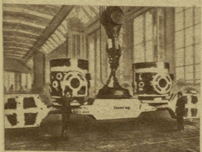
أكبر مقناطيس في العالم حجر المغناطيس الموجود في معامل كروب بألمانيا وقطره ١٥٠٠ مليمتر وهو يحمل ثقل قدره ٧٥ ألف كيلوجرام من الحديد
