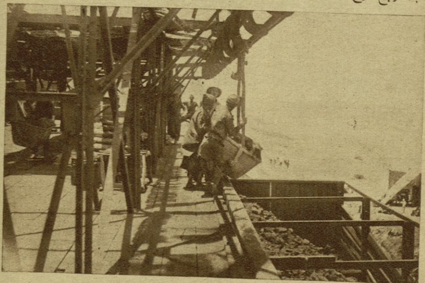
محطة التفريغ عند نهاية الخط الهوائي الذي يصل مناجم أم نجمة بالشاطيء
