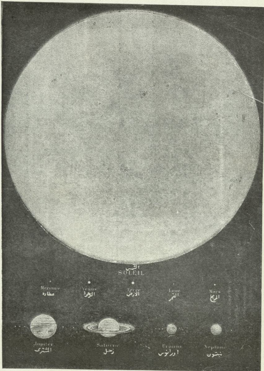
الشمس وبقية السيارات ونسبة اجرامها لبعضها
