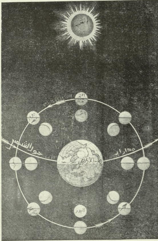
دوران القمر حول الأرض ودوران الأرض حول الشمس
