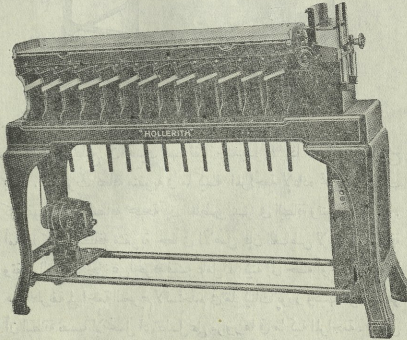
الشكل ٨ . ما كينة الفرز الأفقية
