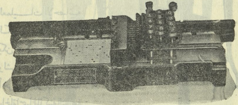
الشكل ٥ . ماكينة التخريم العادية
