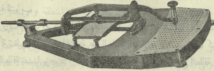
الشكل ٣ . ماكينة التخريم في ١٨٩٠
