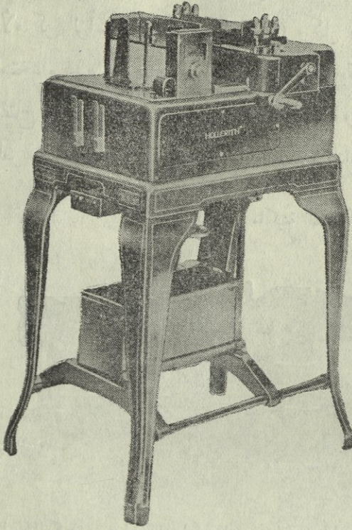
الشكل ٦٠٦ مآكينة التخریم بالجملة
