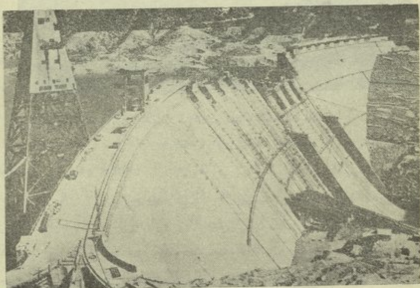
( شكل ٣ ) سد شاستا — منظر جانبي أثناء التثبيت
