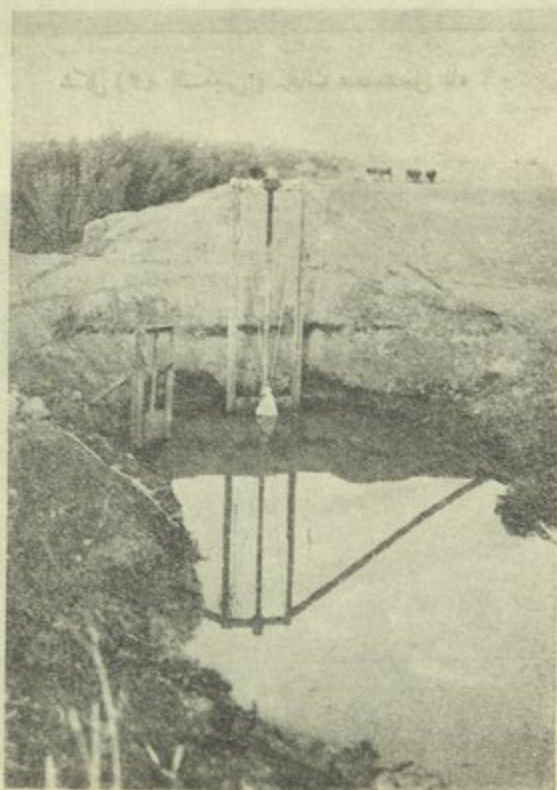
شكل (٢) الكيس بالسلفات وهو معلق على فتحة الحيار
