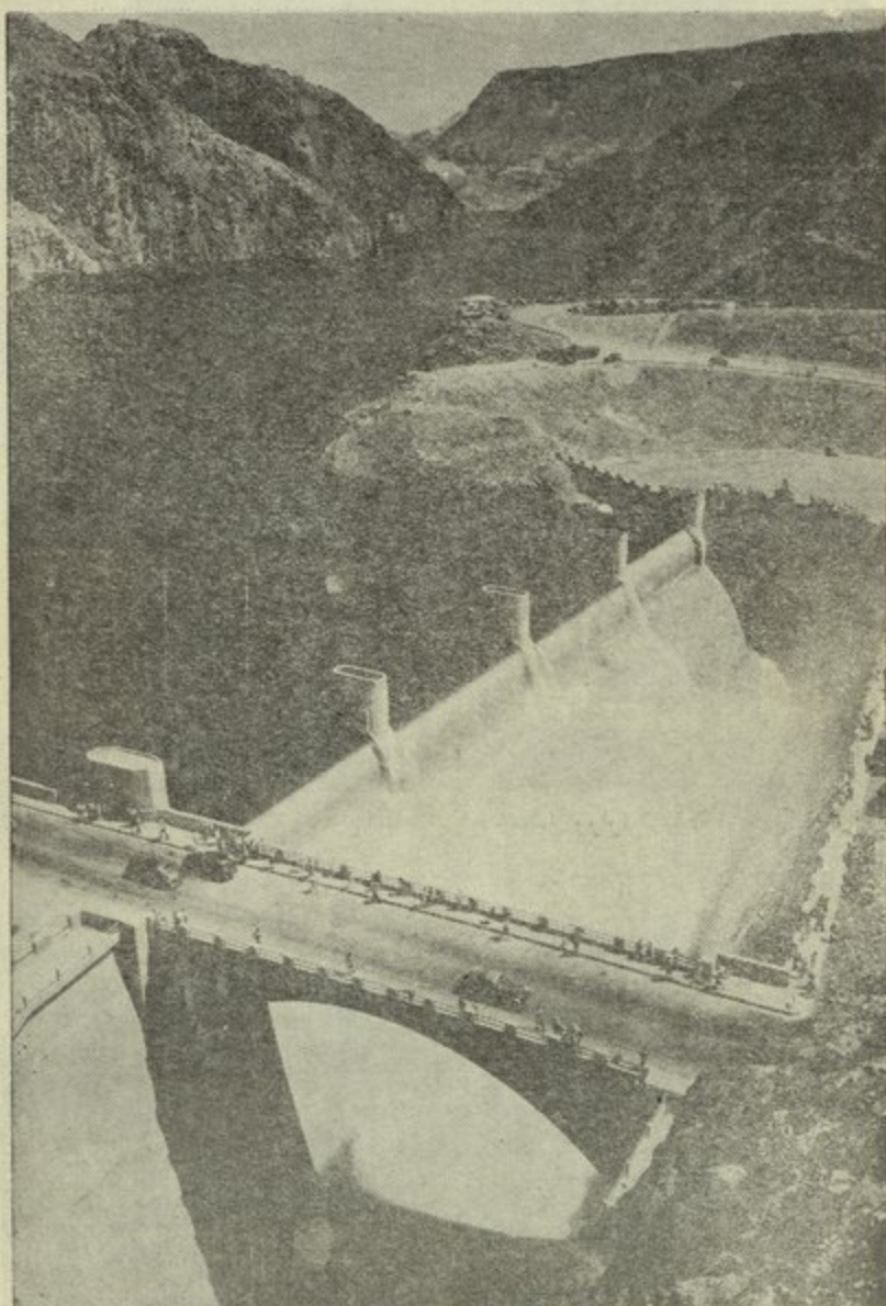
(شكل ١١) سد بولدر - منظر بين شكل الهزار الجانبي
