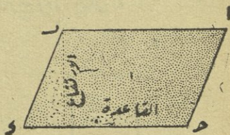
شكل ٥٧ — متوازي الاضلاع
