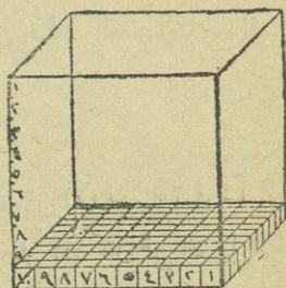
شكل ٦٢ - متر مكعب
