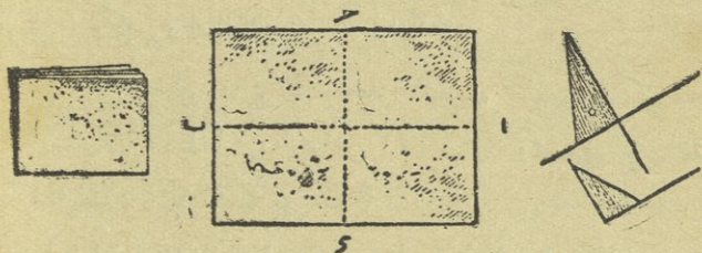
شكل ٢٩ — الخطوط العمودية
