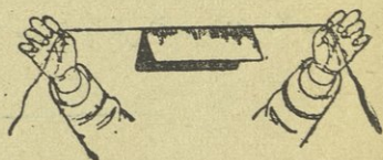
شكل ٦ — الخط المستقيم
