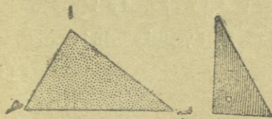
شكل ٥١ — المثلث
