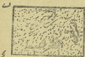
شكل ٤٥ - مستطيل
