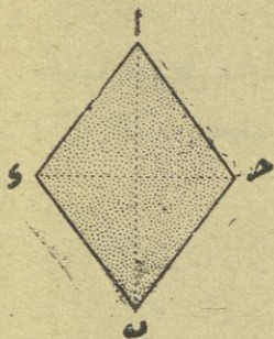
شكل ٥٨ — معين
