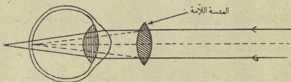
إصلاح قصر النظر بالعدسة المفرقة
