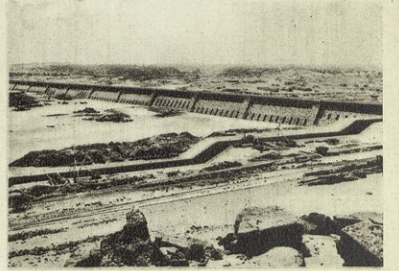
خزان اسوان قبل تعليته
