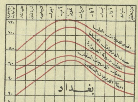
المعدلات الشهرية لدرجات الحرارة في مدينة بغداد مع اوسط اعلی درجة لكل من اشهر السنة خلال مدة 36 سنة.
