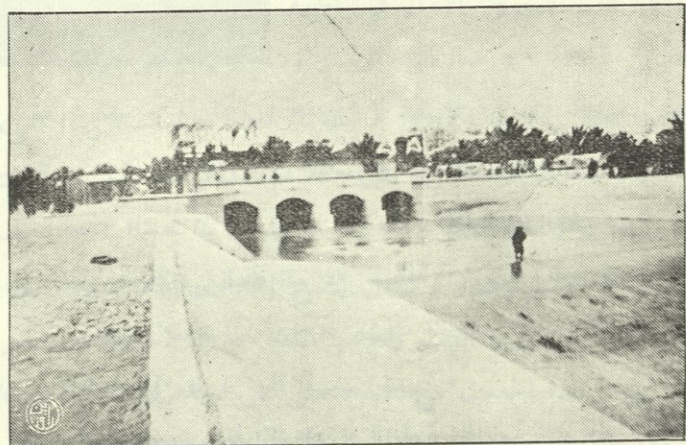
ناظم المشخاب - المنظر من المؤخر
