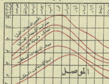
المعدلات الشهرية لدرجات الحرارة في مدينة الموصل مع اوسط اعلی درجة لكل من اشهر السنة خلال مدة 26 سنة.
