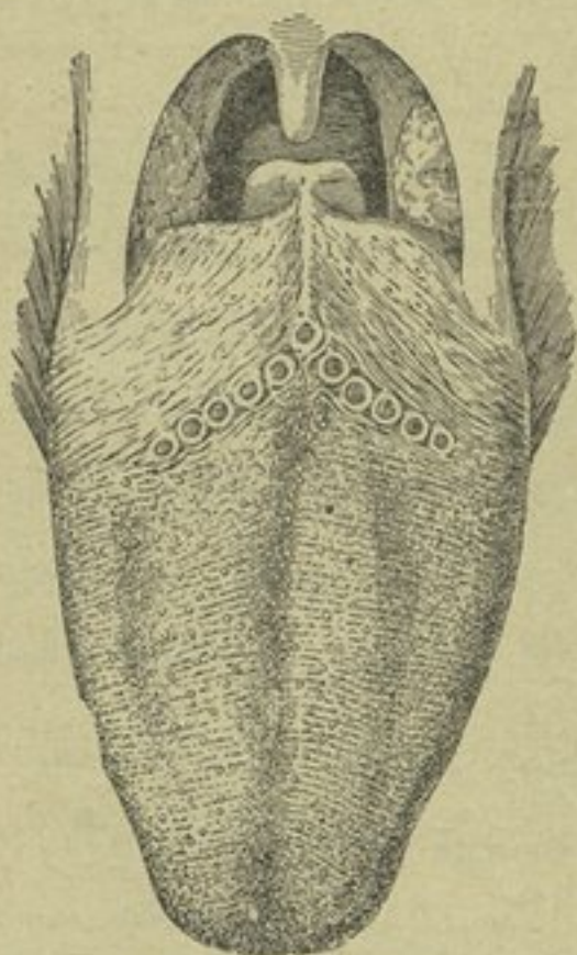
شكل ٣ — عضو الذوق
